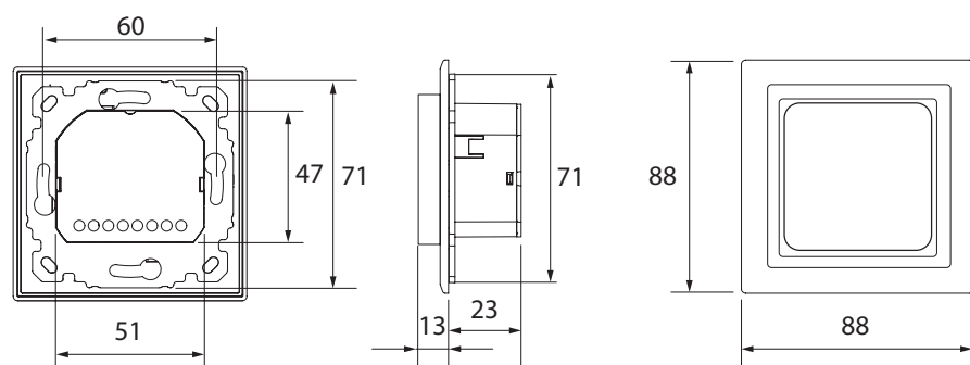
Termostat pokojowy Danfoss Icon ™ 088U1052
